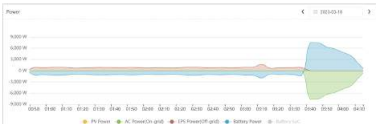
Отрезок времени 16.03 на гибридной ФЭС в Алматы
