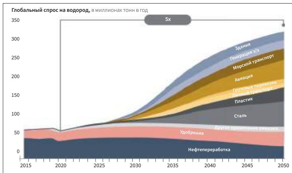
Рисунок 2. Глобальный спрос на водород, в миллионах тонн в год
